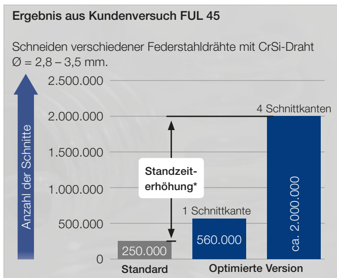
▲ Messerhalter Rotationsschnitt – Arbeitsbeispiel
