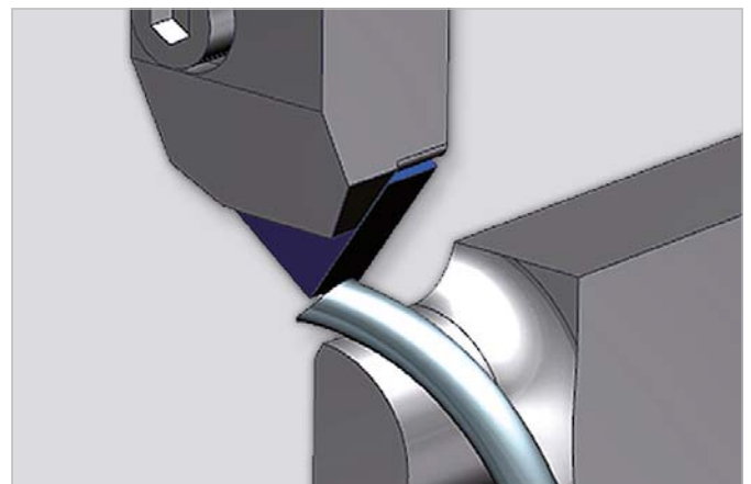
▲ Messerhalter Rotationsschnitt – Arbeitsbeispiel
