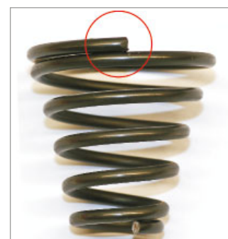
▲ Konische Feder hergestellt mit motorisch verstellbaren Windestifthalter (PTP-Windefinger)
