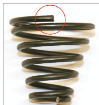
▲ Konische Feder hergestellt ohne motorisch verstellbaren Windestifthalter (PTP-Windefinger)
