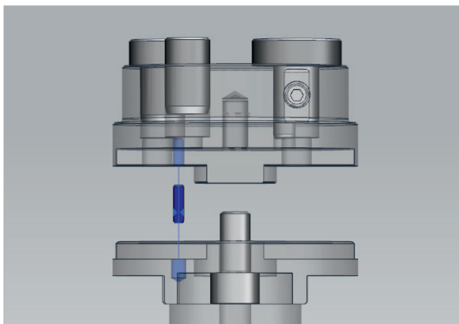
▲ ToolFix Positionierhilfe
