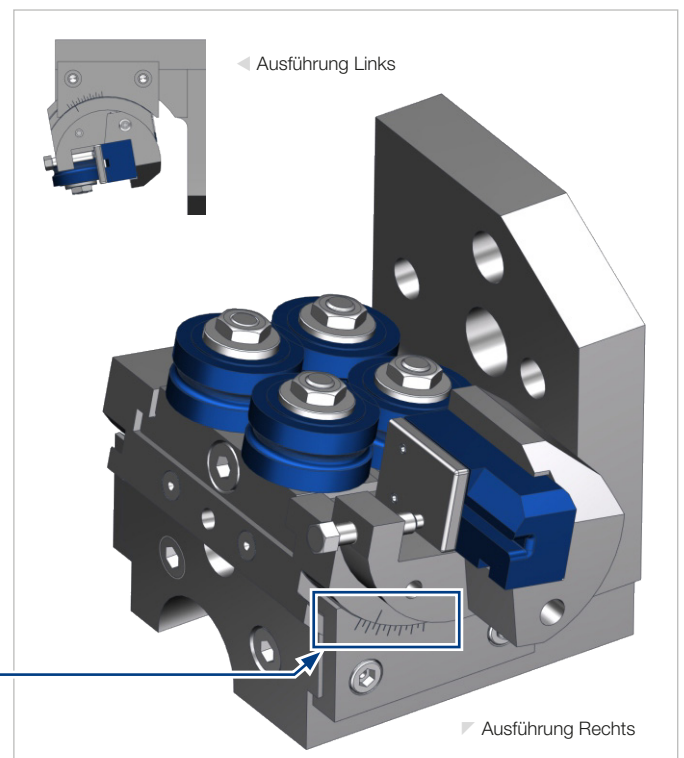
▲ Halter mit drehbarem Windeinsatz - Arbeitsbeispiel
